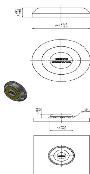
Wzór H (TRID-02/H lub równoważny) – spawany
