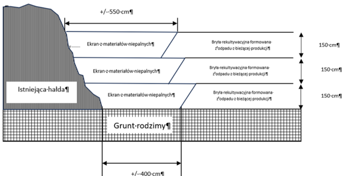
Rys. Schemat wykonania ekranów
