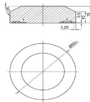
Wzór H (TRID-02/H lub równoważny) – spawany
