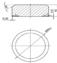
Wzór F (TRID-02/F)
