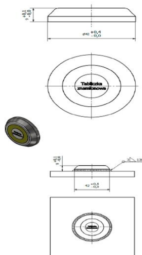
Wzór H (TRID-02/H lub równoważny ) – spawany
