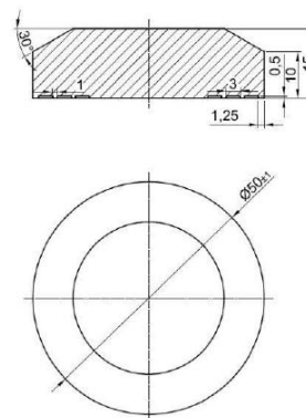
Wzór D (TRID-02/D)
