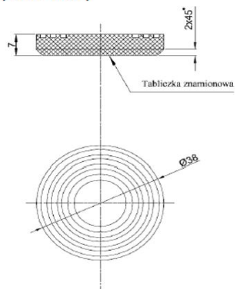
Wzór F (TRID-02/F)
