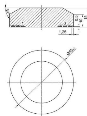
Wzór H (TRID-02/H łub równoważny ) – spawany
