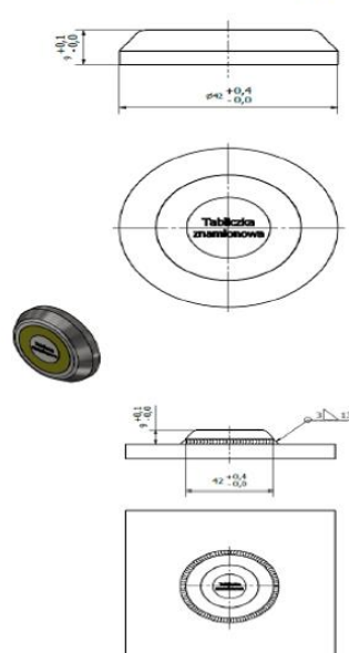
Wzór H (TRID-02/H lub równoważny) – spawany
