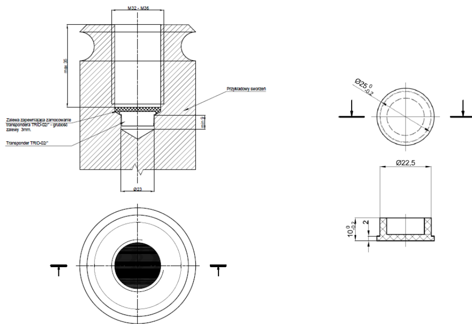
Rysunek montażowy transpondera TRID-02/1 - przykład zabudowy w sworzniu.
