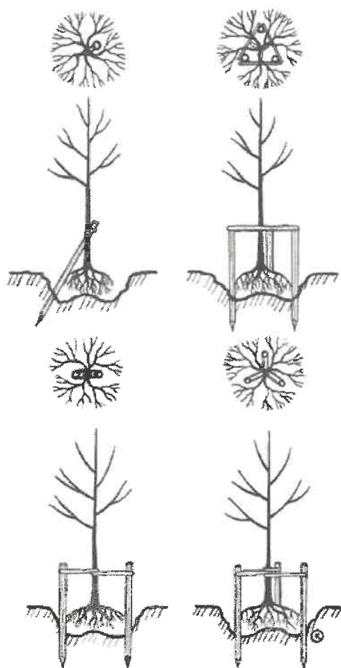
Rysunek 20: Różne rodzaje palikowania.
