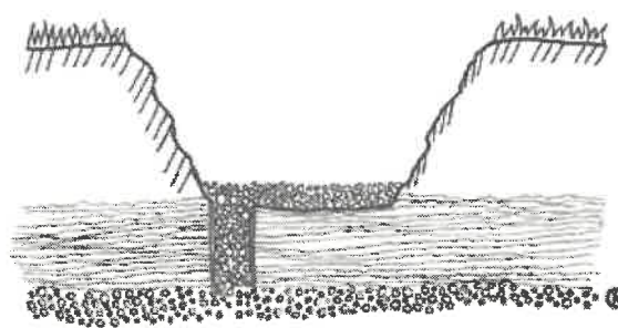
DRENAŻ PIONOWY
