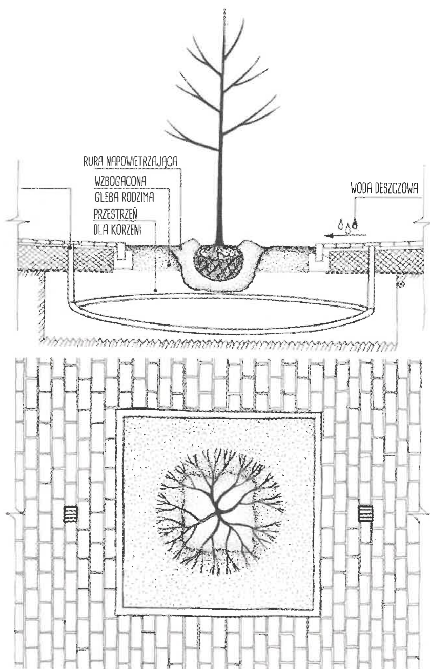
Rysunek 27: Przykładowy system napowietrzania.
