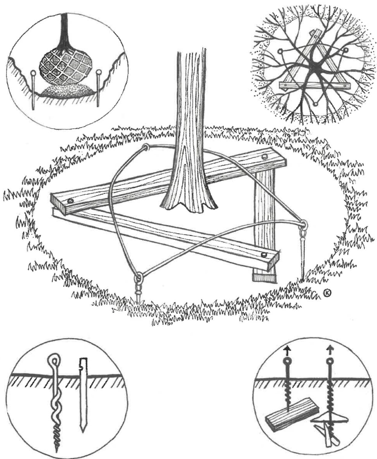
Rysunek 22: Poszczególne elementy podziemnego systemu mocowania.
