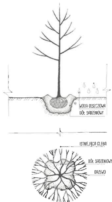
Rysunek 2: Sadzenie drzew w otwartym krajobrazie.
