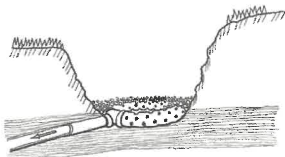
RURA ODWADNIAJĄCA
