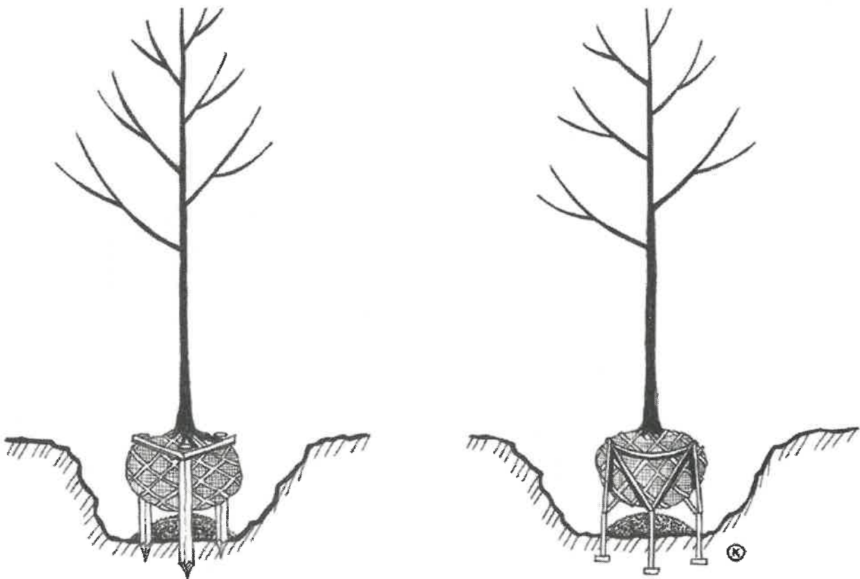
Rysunek 21: Różne rodzaje systemów podziemnego mocowania drzew.
