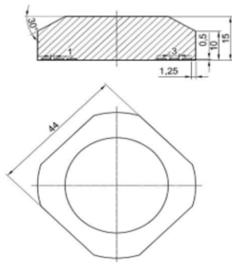
Wzór A (TRID-02/A)
