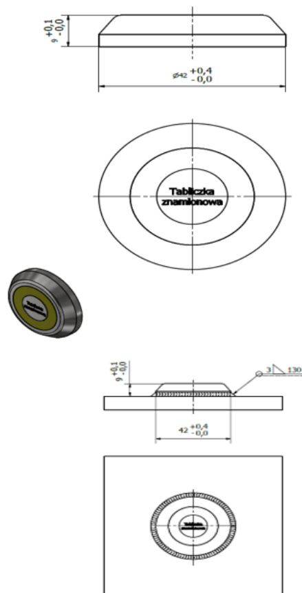
Wzór H (TRID-02/H lub równoważny ) – spawany
