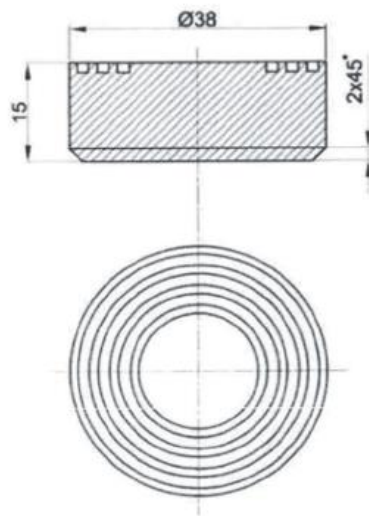
Wzór E (TRID-02/E)
