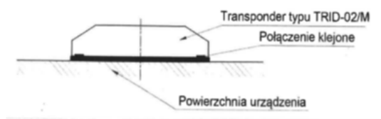
Wzór M (TRID-02/M)
