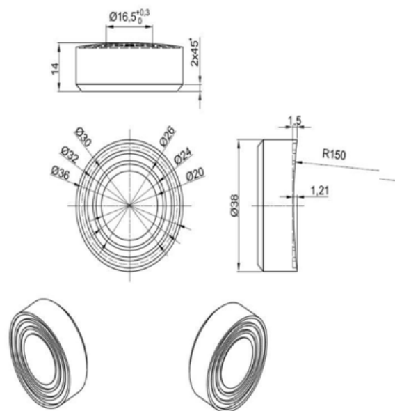
Wzór B (TRID-02/B)
