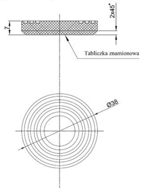
Wzór F (TRID-02/F)
