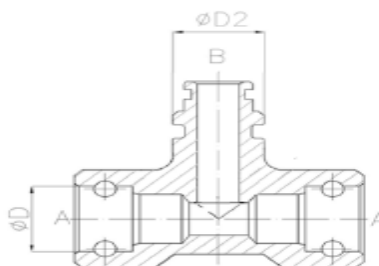
Trójknik typu „T”
